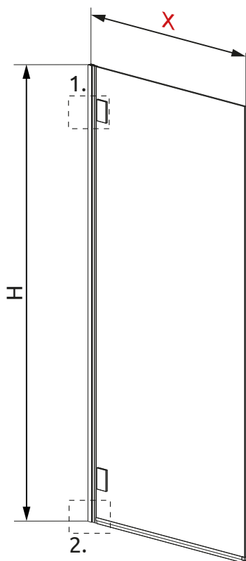
Balos kádparaván Variant L
